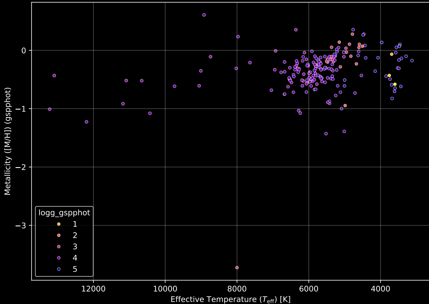
APOGEE DR17 Field: [K2_C7_018-11_btx] Stellar Population Parameters (n= 199)
